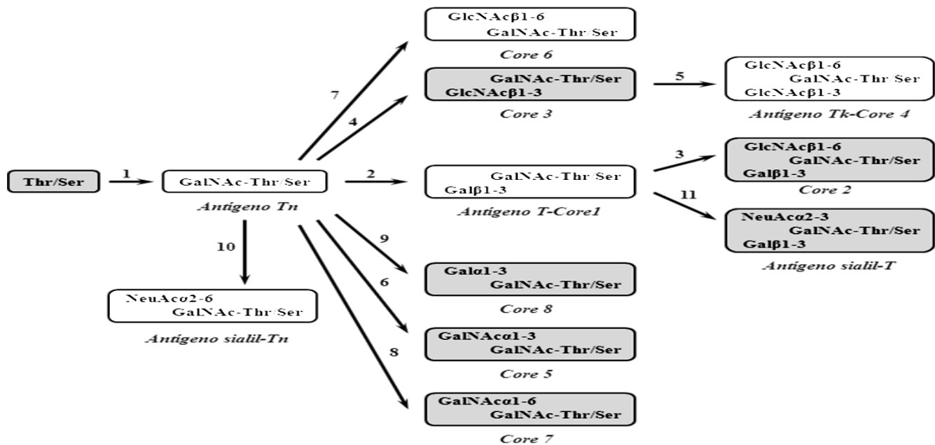
Figura 1. Estructura y biosíntesis del core de los O-oligosacáridos. En color gris claro se indican los principales antígenos asociados a tumor. La primera etapa de la O-glicosilación ocurre por la adición de GalNAc a un residuo de Thr o de Ser de la cadena polipeptídica (paso 1). Ocho tipos diferentes de core pueden formarse por la acción de diversas glicosiltransferasas: core 1 β3Gal-T (paso 2), core 2 β6GlcNAc-T (paso 3), core 3 β3GlcNAc-T (paso 4), core 4 β6GlcNAc-T (paso 5), core 5 α3GalNAc-T (paso 6), core 6 β6GlcNAc-T (paso 7), core 7 α6GalNAc-T (paso 8) y core 8 α3Gal-T (paso 9). Las estructuras sialil-Tn y sialil-T se forman mediante sialilación de los antígenos Tn y T en reacciones catalizadas por la α6-sialil-T (paso 10) o la α3sialil-T (paso 11), respectivamente. Tomado de Freire y col. (2).
